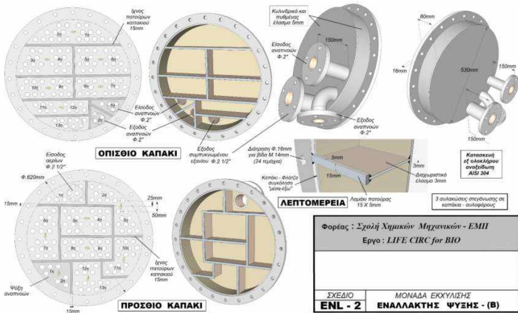
Σχήμα 10. Οπίσθιο και πρόσθιο καπάκι εναλλάκτη ψύξης
