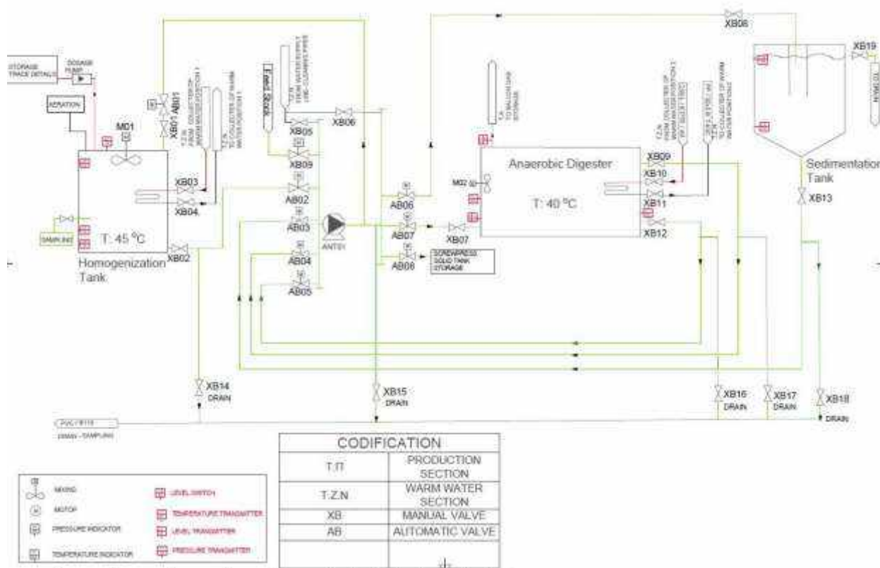
Σχήμα 20. Ηλεκτρική, ηλεκτρονική και υδραυλική διασύνδεση των επιμέρους τμημάτων του πρωτότυπου αναερόβιου χωνευτή δύο σταδίων
