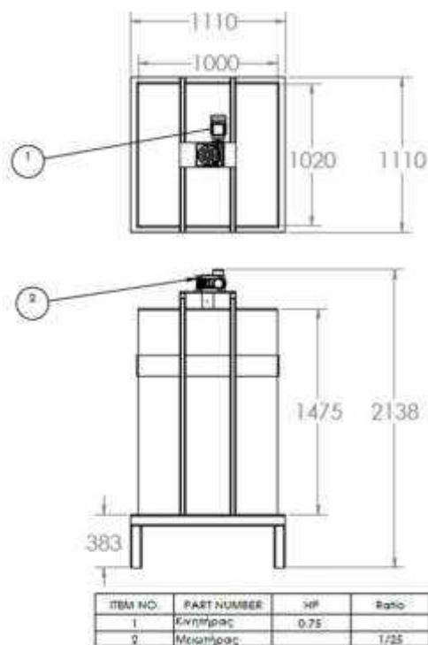
Σχήμα 16. Δεξαμενή ομογενοποίησης
