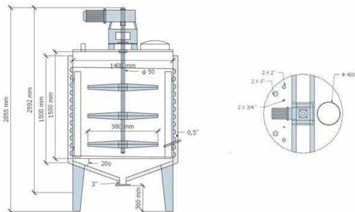
Σχήμα 21. Δεξαμενή θέρμανσης υλικού
