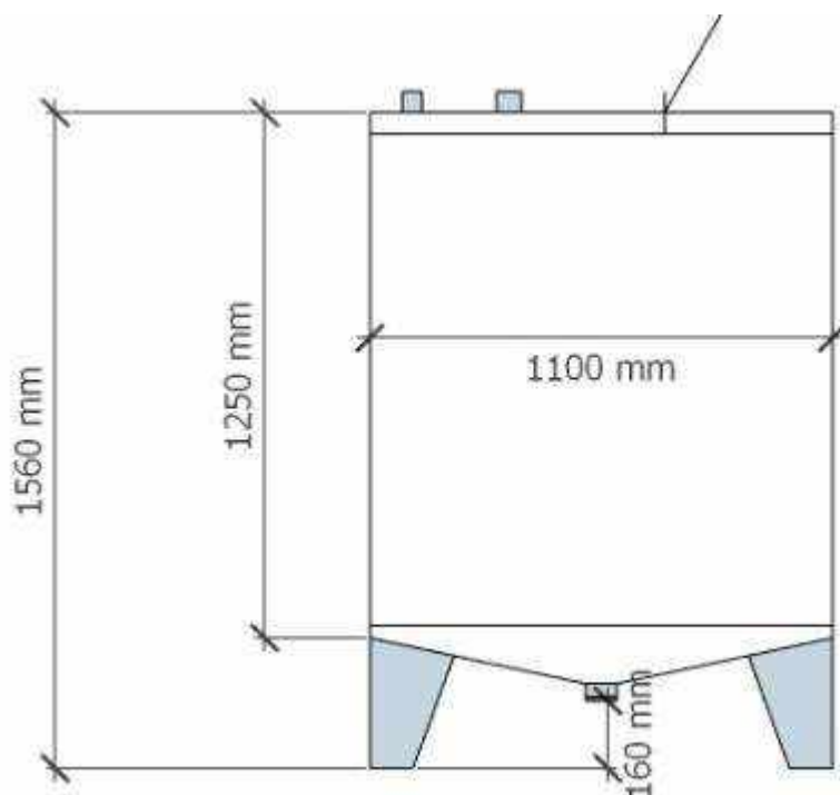
Σχήμα 23. Δεξαμενή αποθήκευσης
