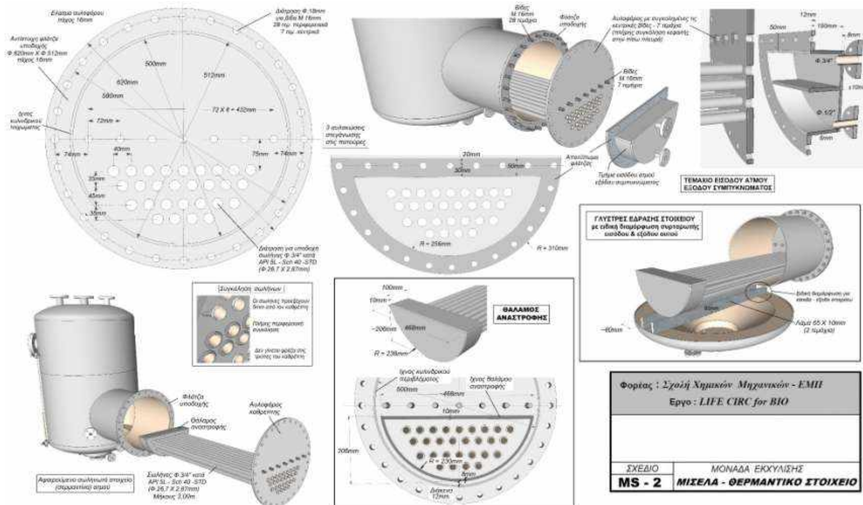
Σχήμα 8. Θερμαντικό στοιχείο της δεξαμενής μισέλας – απόσταξης
