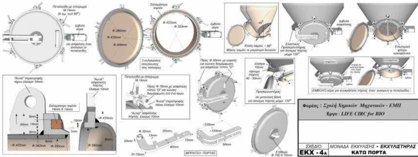
Σχήμα 5. Μονάδα εκχύλισης – Κάτω πόρτα εκχυλιστήρα
