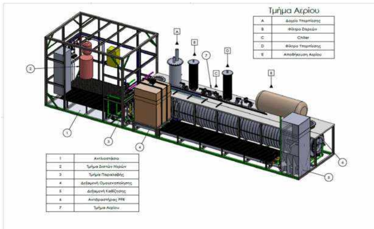
Σχήμα 14. Χωροθέτηση βασικού εξοπλισμού πρωτότυπου αναερόβιου χωνευτή
