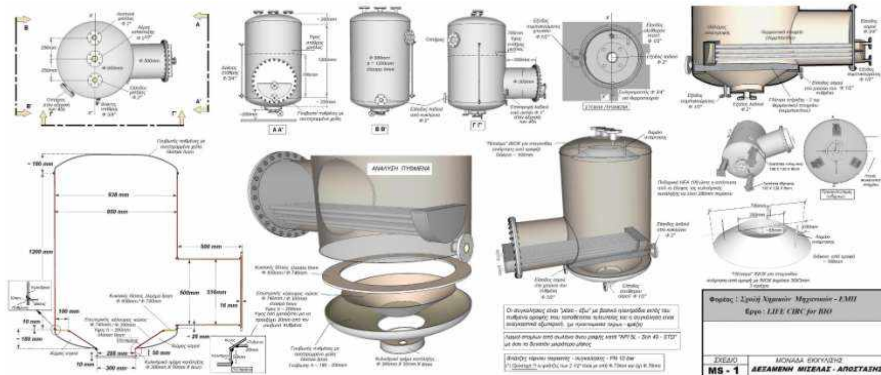
Σχήμα 7. Δεξαμενή μισέλας – απόσταξης
