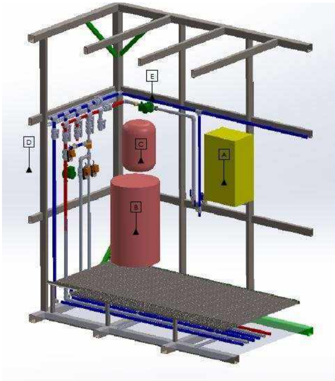
Σχήμα 18. Τμήμα θερμών νερών
