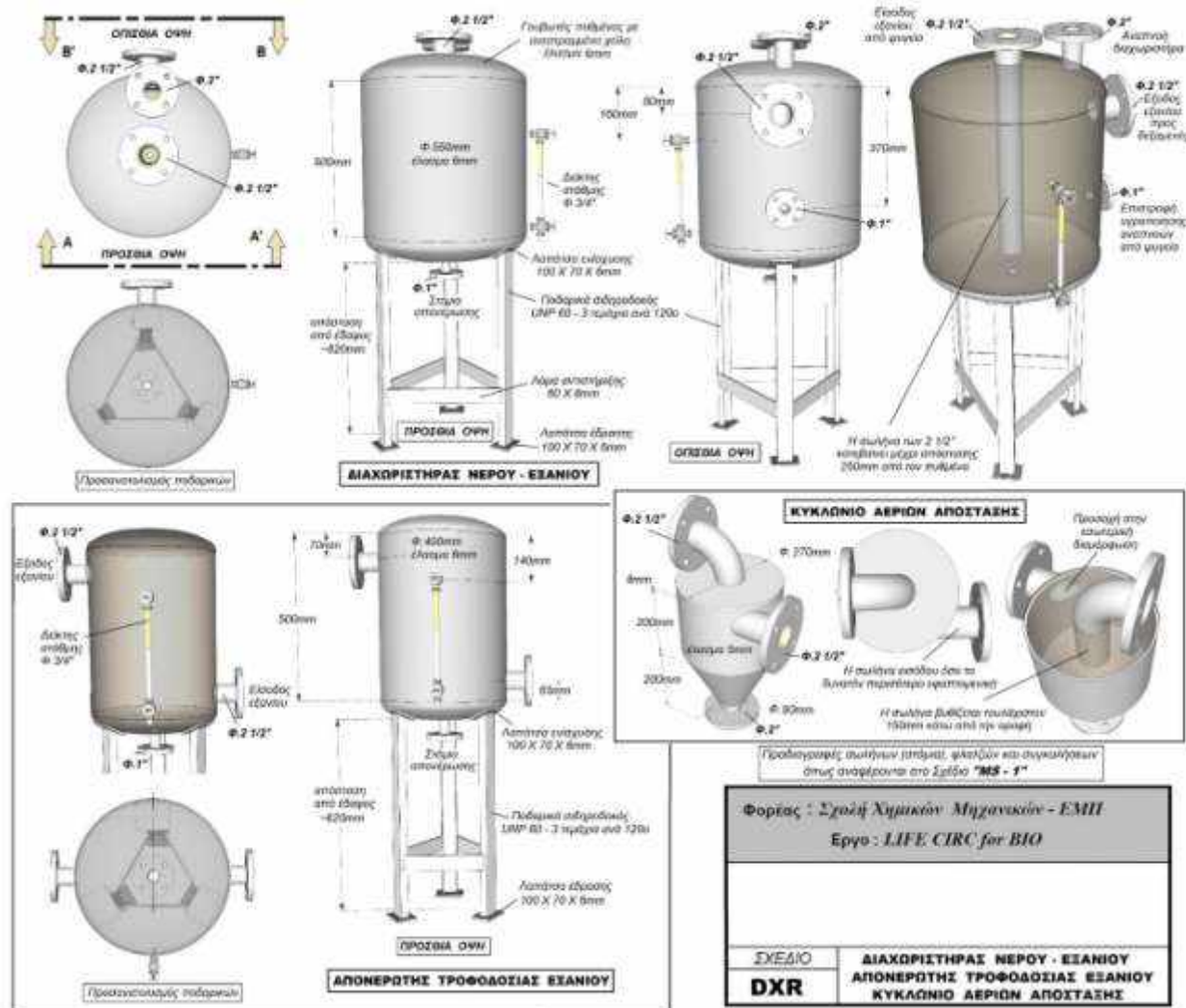
Σχήμα 12. Διαχωριστήρας νερού-εξανίου, απονερώτης τροφοδοσίας εξανίου και κυκλώνιο αερίων απόσταξης
