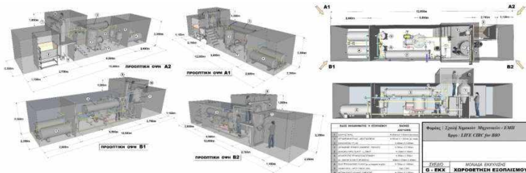
Σχήμα 1. Χωροθέτηση βασικού εξοπλισμού πρωτότυπης μονάδας εκχύλισης με ενσωματωμένο σύστημα για την ανάκτηση και ανακύκλωση του διαλύτη
