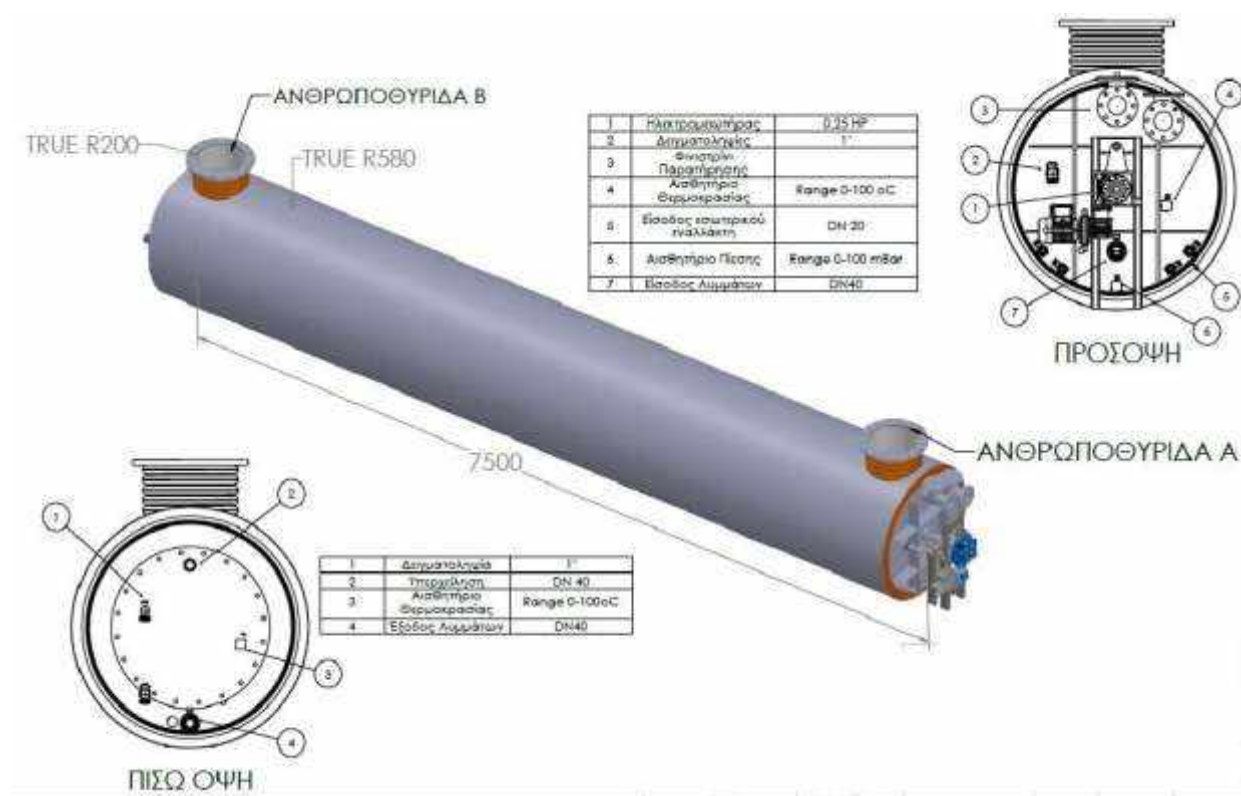
Σχήμα 15. Δεξαμενή βιοαντιδραστήρα
