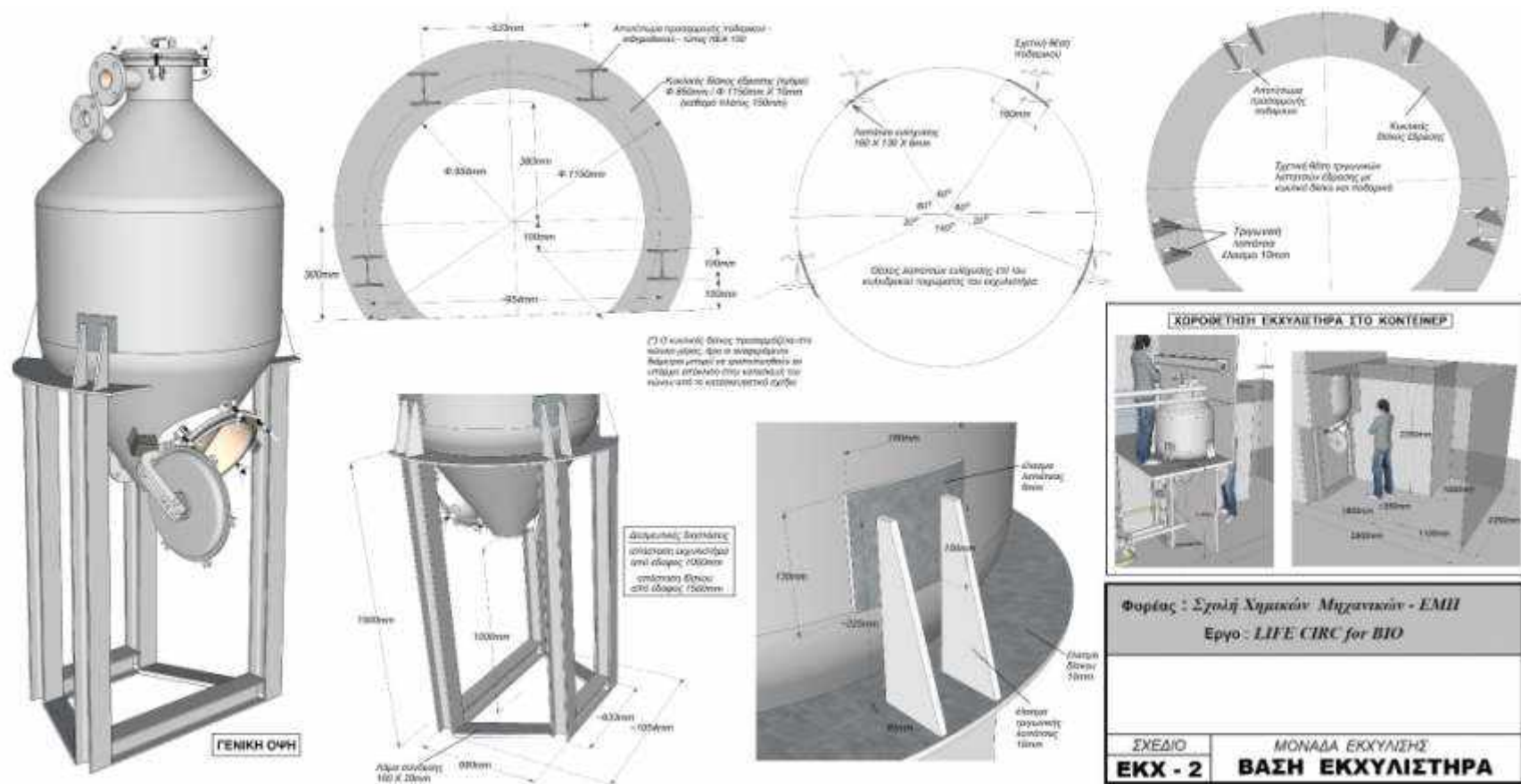
Σχήμα 3. Μονάδα εκχύλισης – Βάση εκχυλιστήρα
