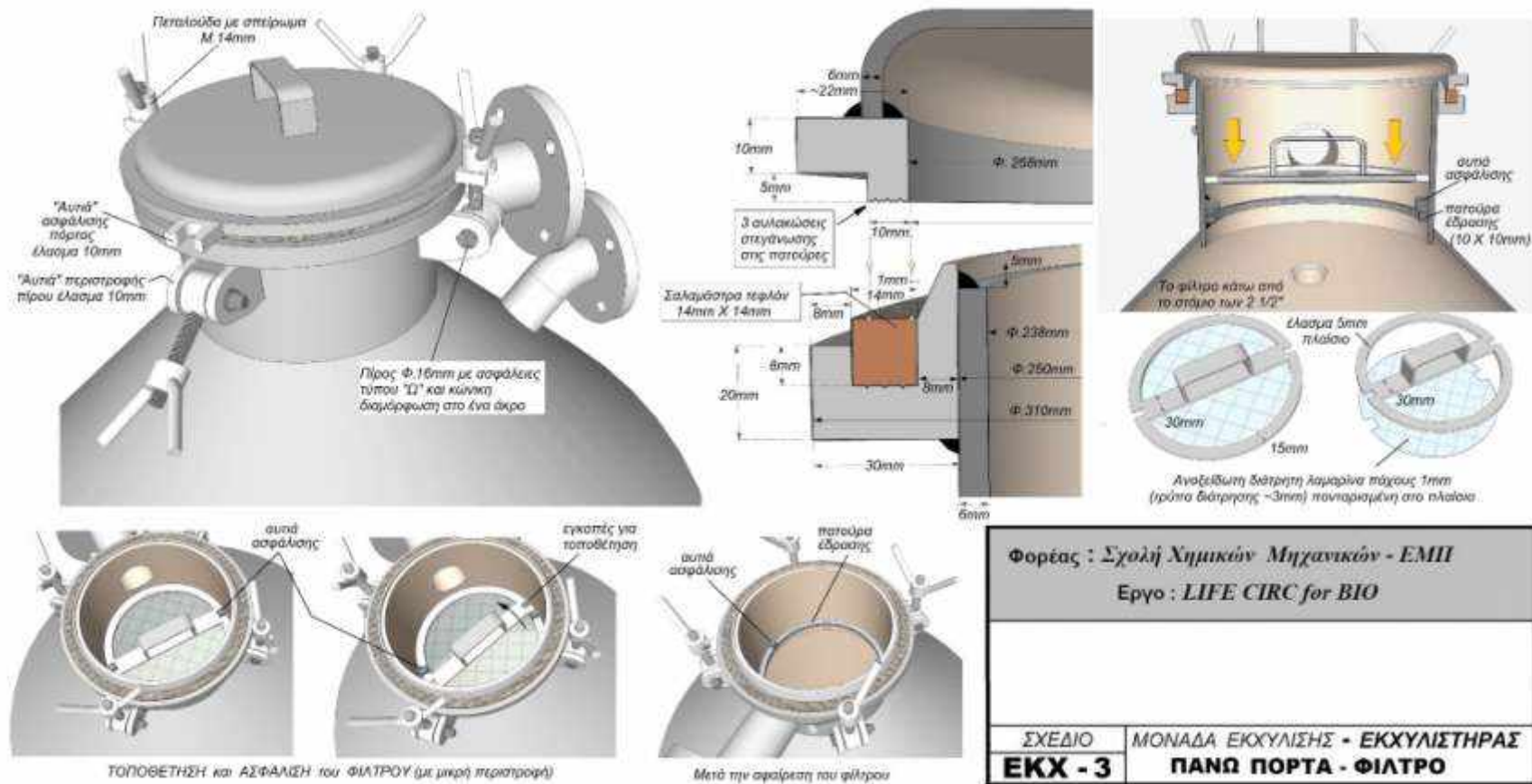
Σχήμα 4. Μονάδα εκχύλισης – Πάνω πόρτα και φίλτρο εκχυλιστήρα
