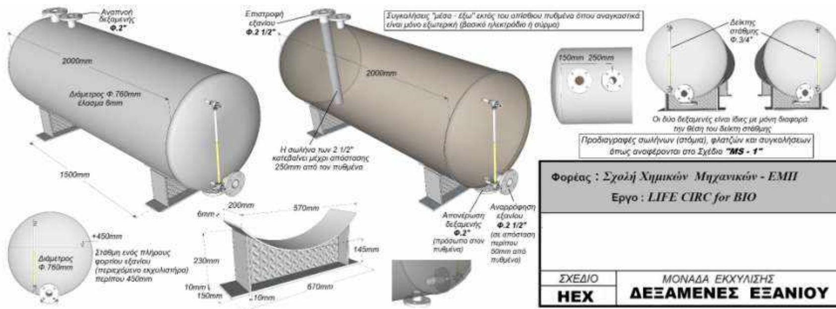
Σχήμα 11. Δεξαμενές εξανίου
