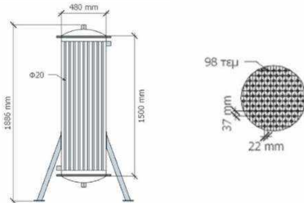
Σχήμα 22. Συμπυκνωτής
