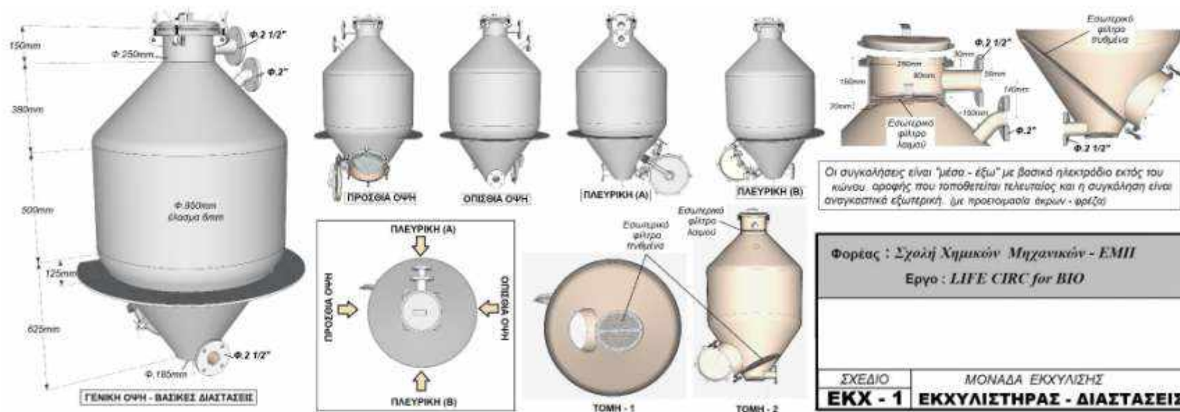
Σχήμα 2. Μονάδα εκχύλισης – Διαστάσεις εκχυλιστήρα
