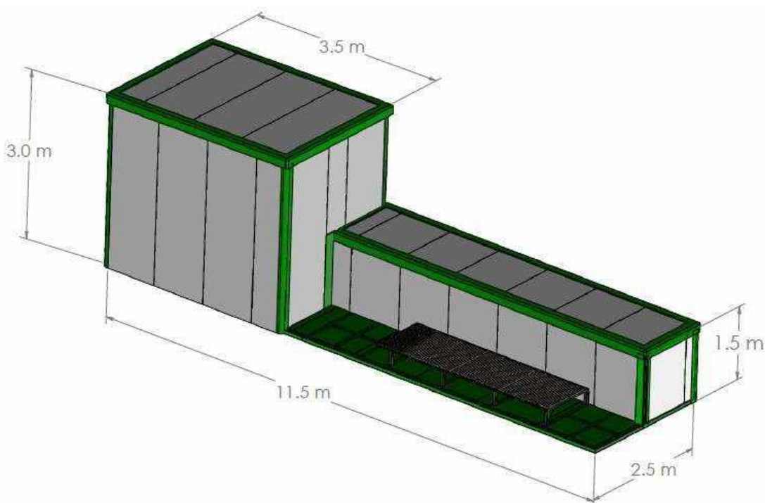
Σχήμα 13. Διαστάσεις και σχήμα κατασκευής πάνελ για τον πρωτότυπο αναερόβιο χωνευτή
