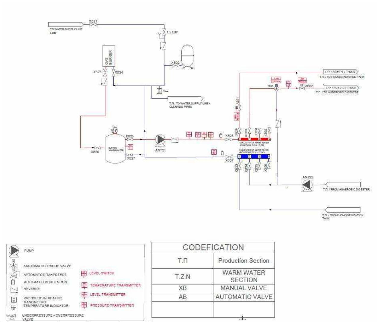
Σχήμα 19. Διάγραμμα τμήματος θερμών νερών
