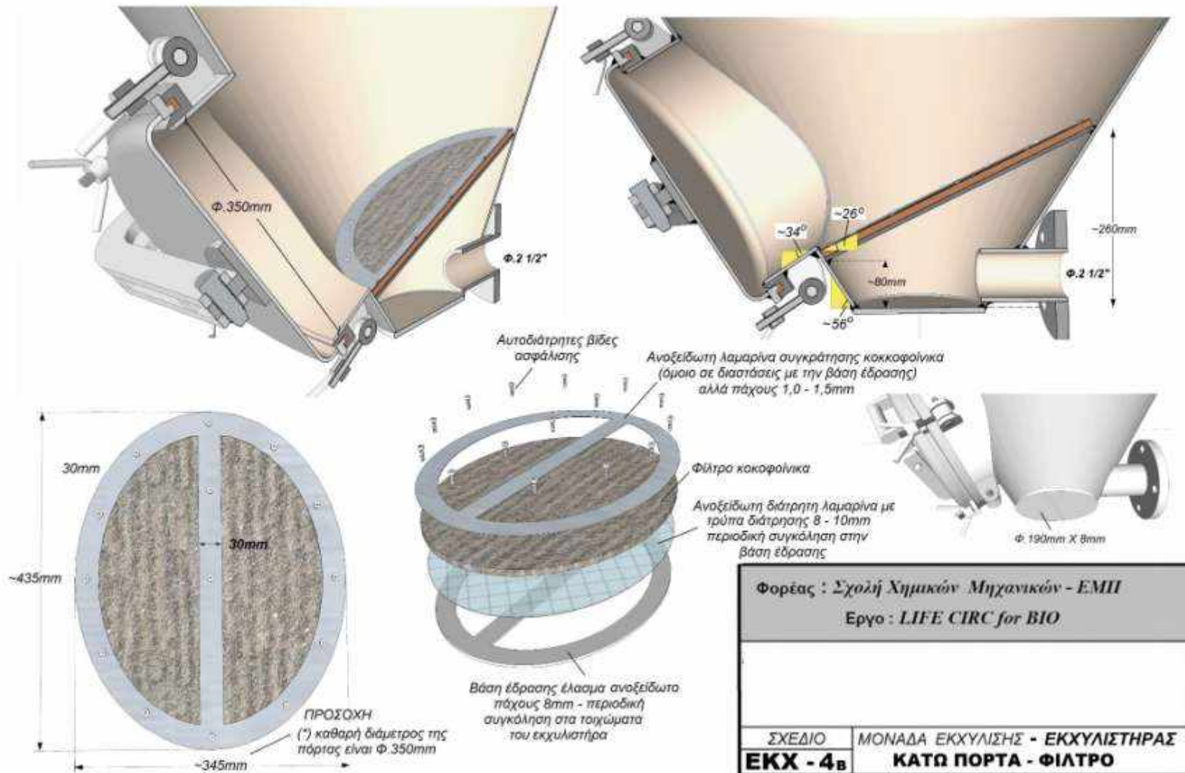
Σχήμα 6. Μονάδα εκχύλισης – Κάτω πόρτα και φίλτρο εκχυλιστήρα
