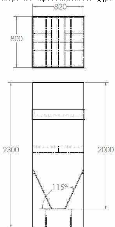
Σχήμα 17. Δεξαμενή καθίζησης
