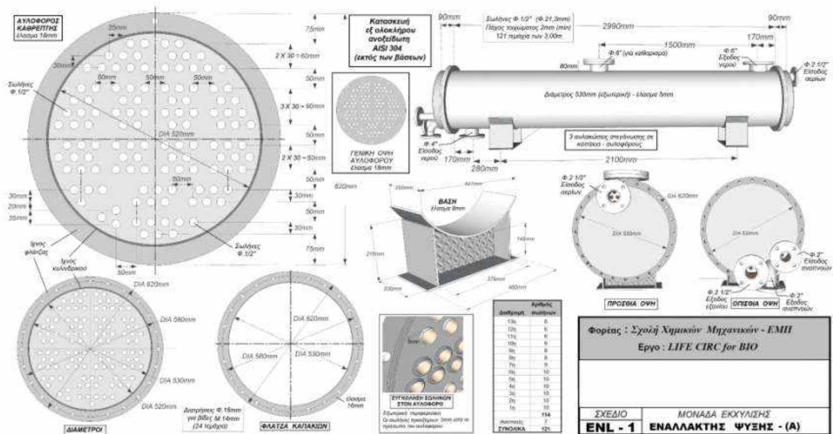
Σχήμα 9. Εναλλάκτης ψύξης
