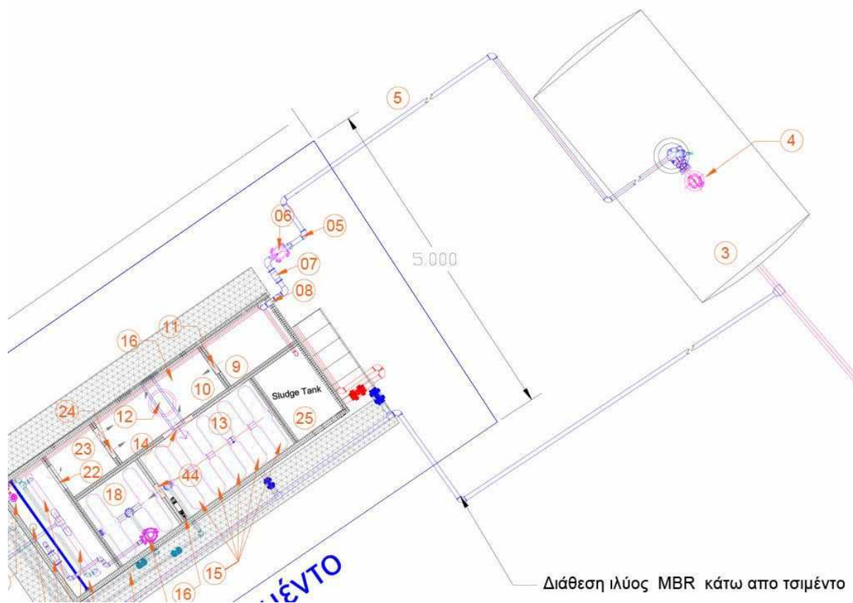
Σχήμα 2: Δεξαμενή Buffer τροφοδοσίας και δεξαμενές βιολογικής επεξεργασίας (Κάτοψη)
