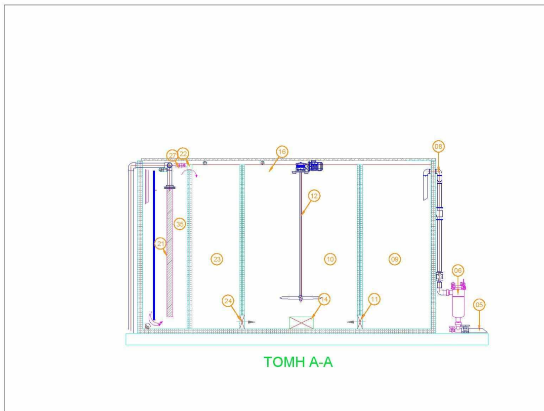
Σχήμα 4: Δεξαμενές βιολογικής επεξεργασίας (Τομή)
