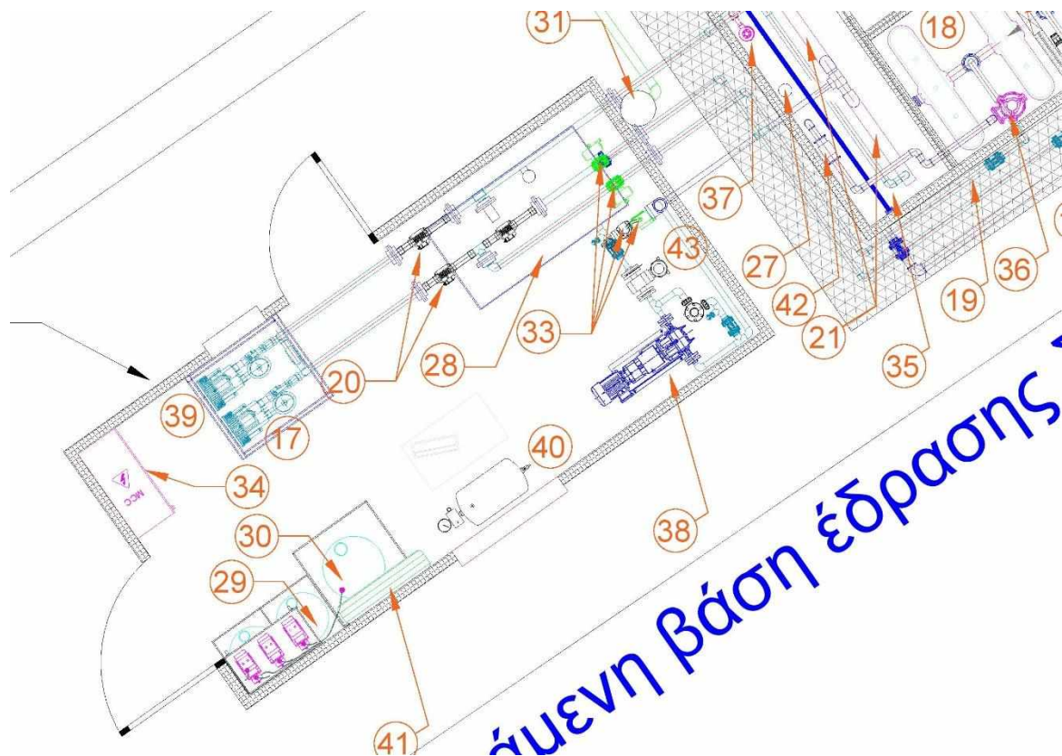
Σχήμα 6: Οικίσκος Ηλεκτρομηχανολογικού εξοπλισμού (Container machine room, Κάτοψη)
