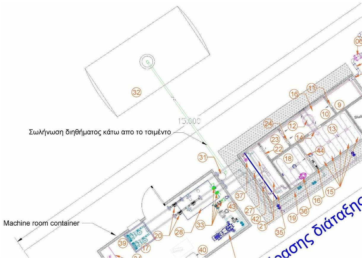
Σχήμα 7: Δεξαμενή διήθηματος και δεξαμενές βιολογικής επεξεργασίας (Κάτοψη)
