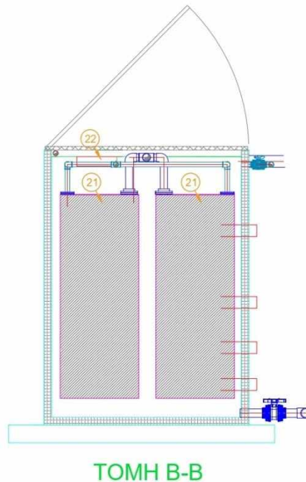
Σχήμα 3: Δεξαμενή εμβαπτισμένων μεμβρανών Υπερδιήθησης (Τομή)
