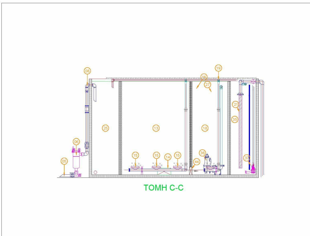
Σχήμα 5: Δεξαμενές βιολογικής επεξεργασίας (Εναλλακτική Τομή)
