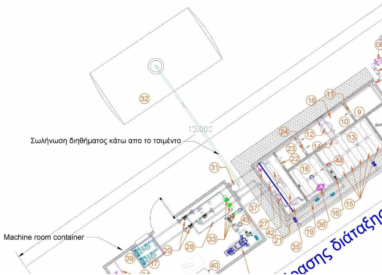
Σχήμα 7: Δεξαμενή διηθήματος και δεξαμενές βιολογικής επεξεργασίας (Κάτοψη)
